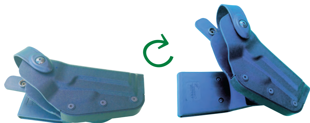
Art. prgh Passante che permette una rotazione a 360° delle nostre fondine + art. ab1 Arco di sicurezza livello I per estrazione rapida + art. 1fpo fondina in pelle e polimero iniettato
